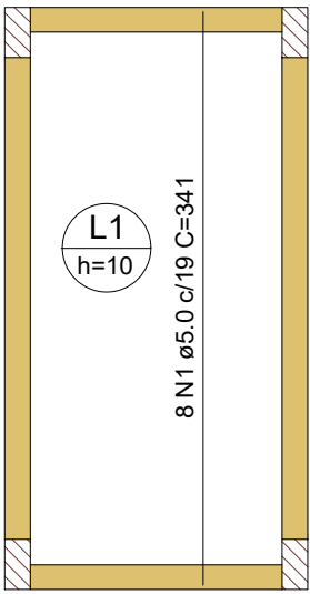
Armação positiva das lajes do pavimento +380 (Eixo Y) escala 1:50
