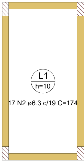
Armação positiva das lajes do pavimento +380 (Eixo X) escala 1:50
